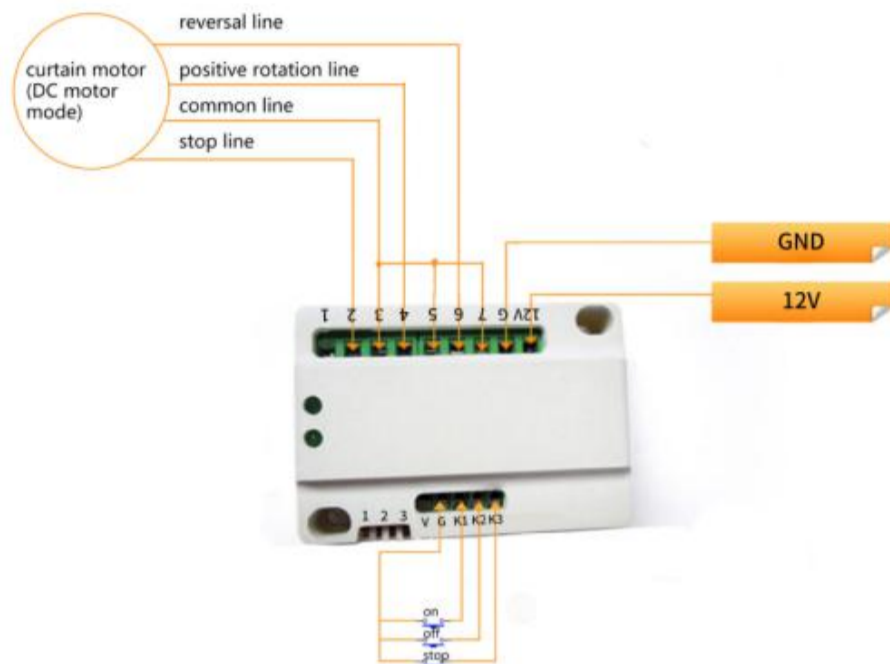
接线图
